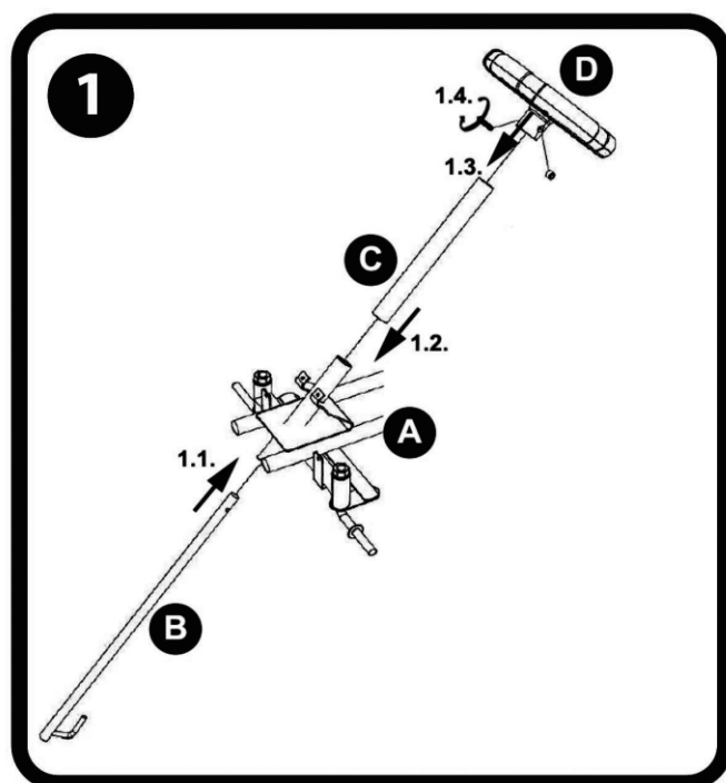
1. Ensemble de la tige de direction et du volant
