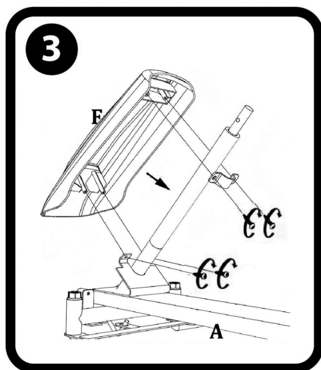
3. Montaggio del pannello frontale
