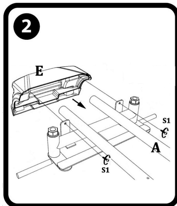
2. Assemblage de la partie avant de la tête
