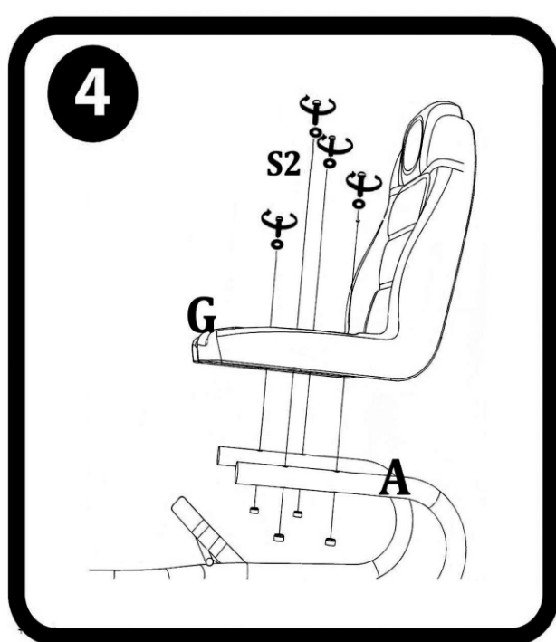
4. Sitzanordnung
