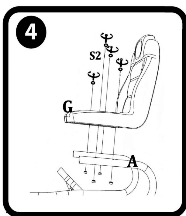
4. Assemblage du siège
