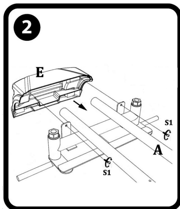
2. Assemblaggio della parte anteriore della testa
