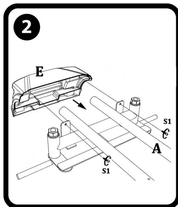
2. Montagem da parte frontal da cabeça
