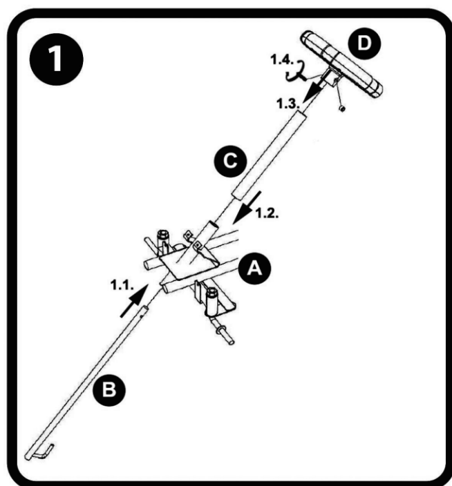
1. Conjunto de barra de dirección y volante
