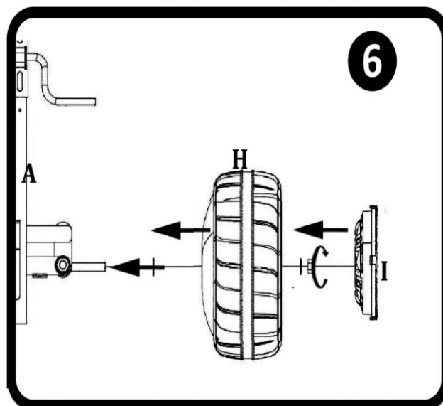
6. Assemblaggio delle ruote anteriori (2 lati)
