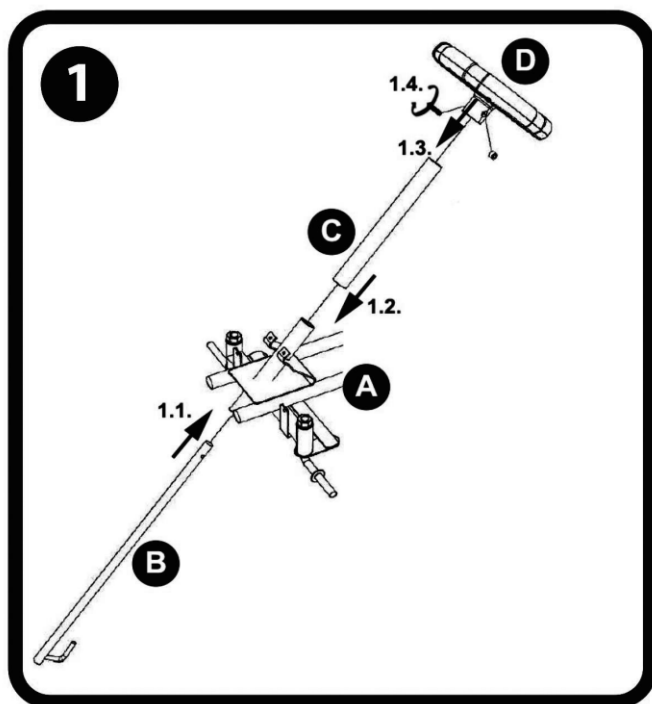
1. Lenkstock + Lenkrad-Set
