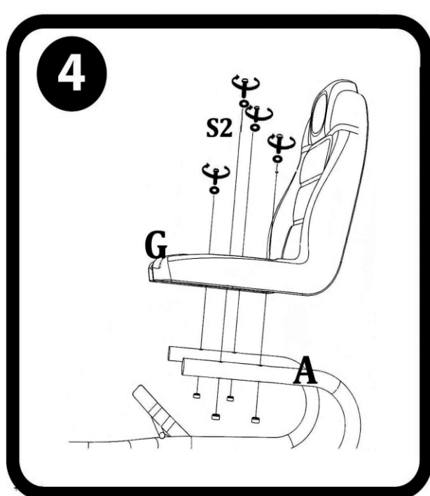
4. Assemblaggio del sedile
