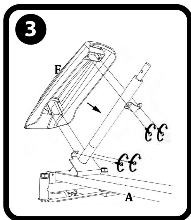
3. Asamblarea panoului frontal
