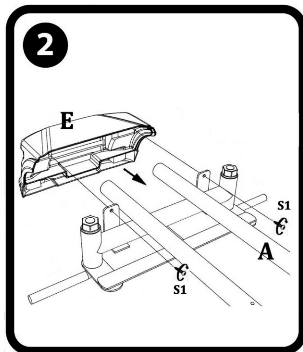
2. Montage des vorderen Kopfbereichs
