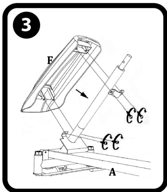
3. Montage des Vorderpaneels
