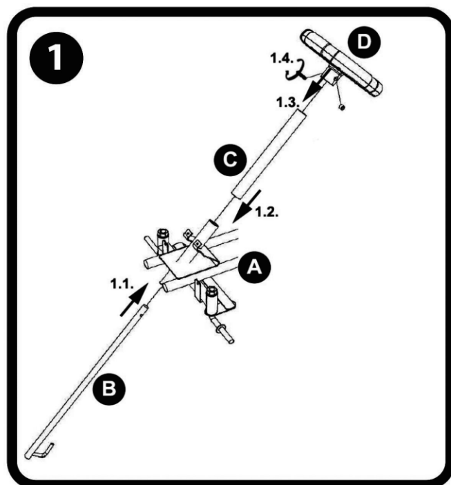
1. Ensemble de la tige de direction et du volant
