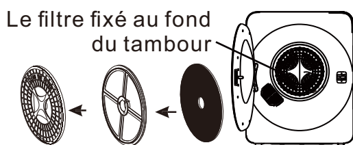
Couvercle de la sortie d'air Filtre à peluches Filtre d'échappement
