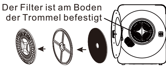
Der Filter ist am Boden der Trommel befestigt Abluftabdeckung Flusenfilter Abluftfilter Abbildung 1
