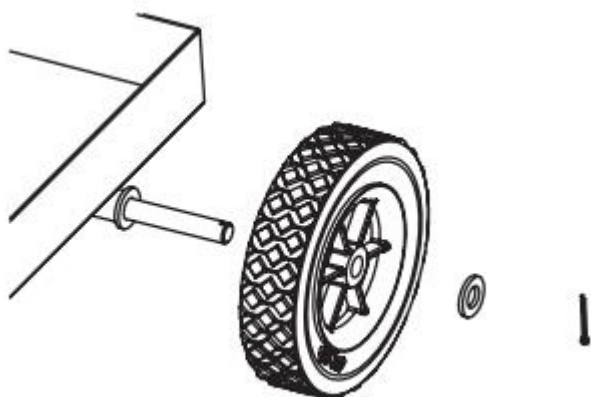
Figure A : Fixation de la roue
