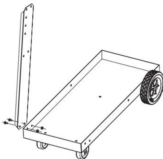
Figura C: Conexión de la Estantería Inferior y el Soporte Izquierdo
