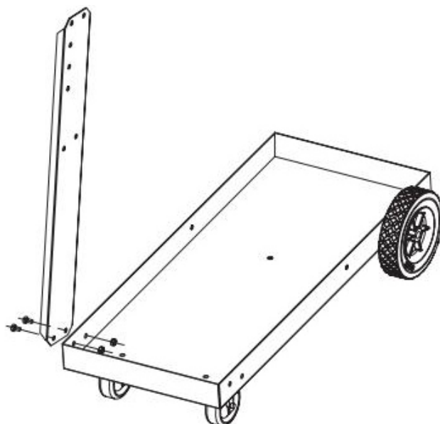
Figure C : Connexion de l'étagère inférieure et du support gauche
