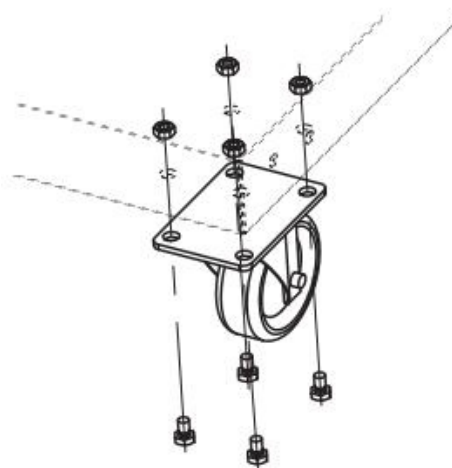
Figura B: Montaggio delle ruote
