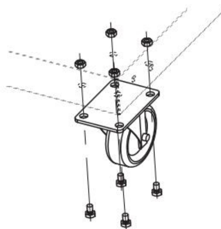
Figure B : Fixation du rouleau pivotant
