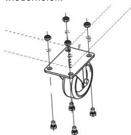
Abbildung B: Rollenbefestigung
