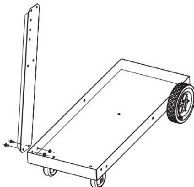
Abbildung C: Verbindung von unterem Regal und linker Stütze
