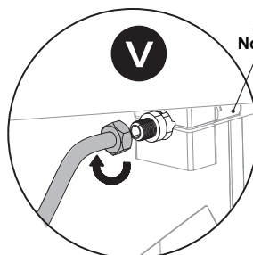
Install the corrugated gas hose Installer le tuyau d'alimentation gaz ondulé.
