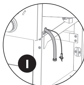
Thread through the grill body hole Passer à travers l'orifice du corps du gril.
