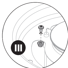
Attach with an M4x8mm [F] screw and an M4 nut [G] Fixer à l'aide d'une vis M4x8 mm [F] et d'un écrou M4 [G].
