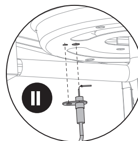
Thread through the side burner body hole Passer à travers l'orifice du corps du brûleur latéral.
